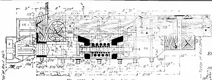
Fig. 1959. Longitudinal Section.
